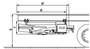
Montage semi-remorque avec plate-forme 1 fois repliée
