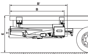
Montage porteur avec plate-forme 1 fois repliée
