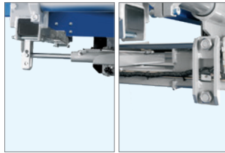
Double vérin de rétraction boulonné avec fixation boulonnée au véhicule
