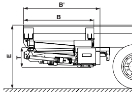
Montage porteur avec plate-forme 2 fois repliée
